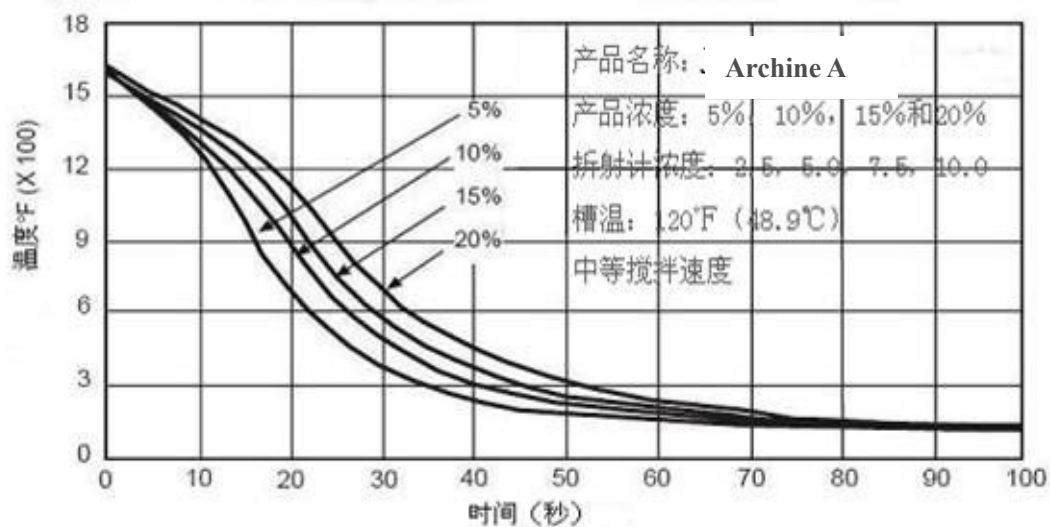
图表2 槽温升高对冷却率的影响
